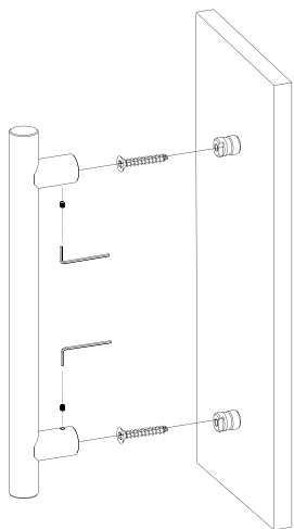
MONTAŻ POCHWYTU JEDNOSTRONNEGO NA DREWNOWKRĘT SINGLE PULL HANDLE ASSEMBLY WITHOUT HOLES
