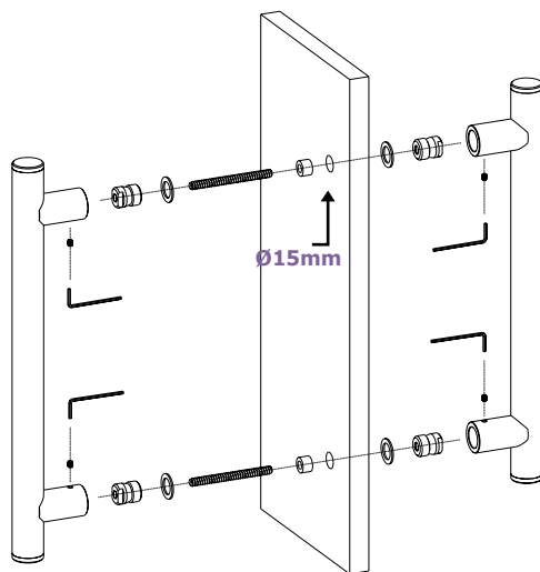
MONTAŻ POCHWYTU DWUSTRONNEGO DO DRZWI SZKŁANYCH PAIR PULL HANDLES ASSEMBLY IN GLASS
